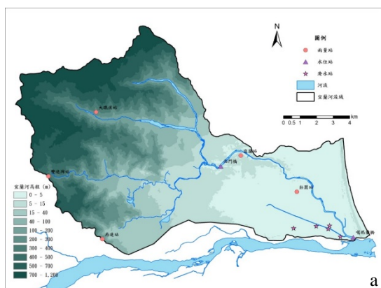
圖 6 宜蘭河試驗流域內用以推估流量之測站佈置
