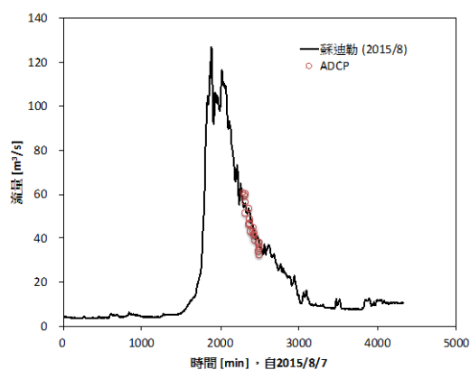
圖 8 宜蘭河員山大橋站於蘇迪勒颱風期間：a 現場流況與觀測作業情況；b 觀測流量與推估流量比較結果
